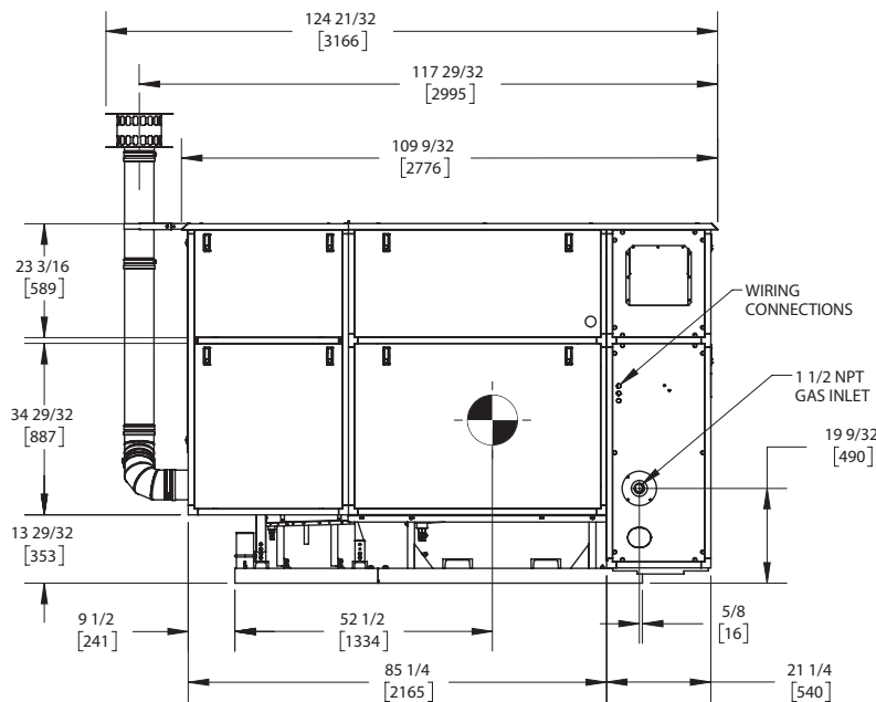
SIDE VIEW ASUB-00065_B
